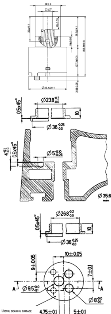
limitatore temperatura LT adjustable temperature limiter LT limitatore di portata LP adjustable flow rate limiter LP
