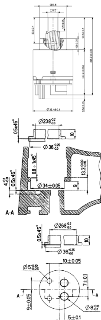
limitatore temperatura LT adjustable temperature limiter LT limitatore di portata LP adjustable flow rate limiter LP
