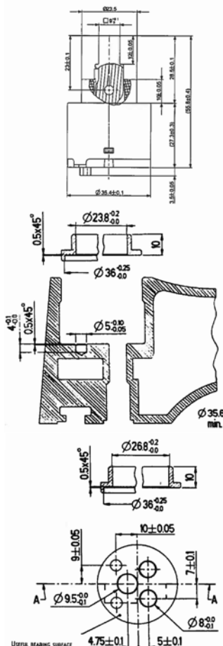
limitatore di portata e temperatura LPT adjustable flow rate and temperature limiter LPT
