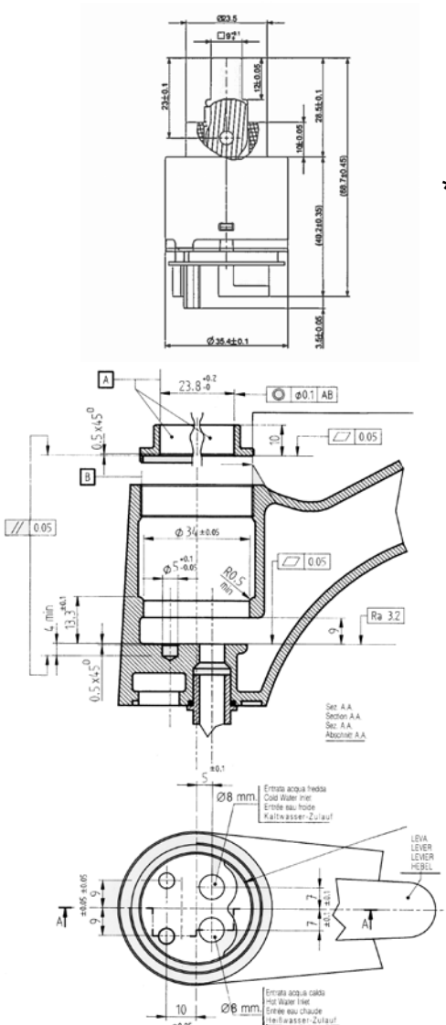
limitatore di portata e temperatura LPT adjustable flow rate and temperature limiter LPT
